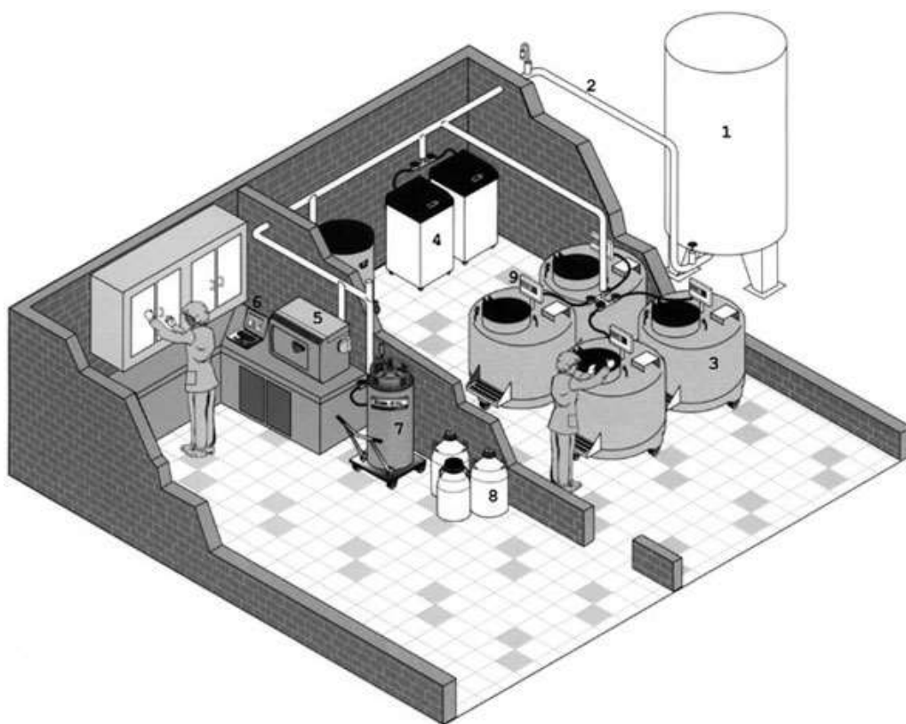
Рис. 15.7. Схема помещений и оборудования криобанка
