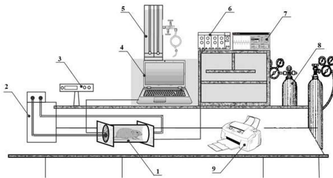
Рис. 22.1. Схема компьютеризированной установки для программного охлаждения и разогрева лабораторных животных. 1 – холодная камера с водяной рубашкой для животных, 2 – охлаждающий термостат, 3 – дисплей температуры, 4 – компьютер, 5 – система контроля газового потока, 6 – блок управления, 7 – осциллограф, 8 – баллоны с дыхательной смесью, 9 – принтер.
