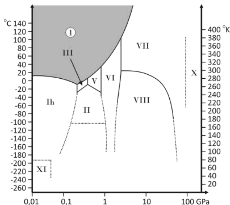
Рис. 4.7. Фазовая диаграмма льда. Давление (ГПа) в логарифмическом масштабе, температура слева — в градусах Цельсия, справа — Кельвина, 1 — жидкая фаза.
