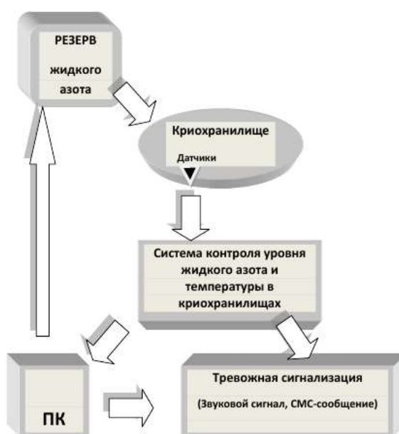
Рис. 15.6. Схема контроля и пополнения криохранилищ жидким азотом. С датчика температуры, расположенного внутри криохранилища, постоянно передаётся информация на системный блок и затем на персональный компьютер. После обработки сигнала, в случае недопустимого снижения уровня азота внутри хранилища, включается тревожная сигнализация и из резервной ёмкости начинает поступать жидкий азот.
